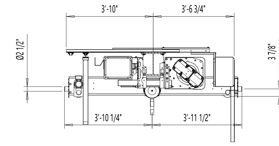
View A-A
