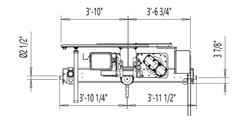
View A-A
