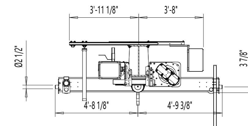
View A-A
